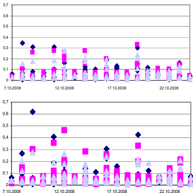
Obr. 3 Grafy maximálních rychlostí kmitání (v \text{mm}\cdot\text{s}^{-1} ) naměřených na stanicích KAR A, KAR B a KAR C; nahoře vertikální složky, vlevo dole horizontální N-S složky, vpravo dole horizontální E-W složky
